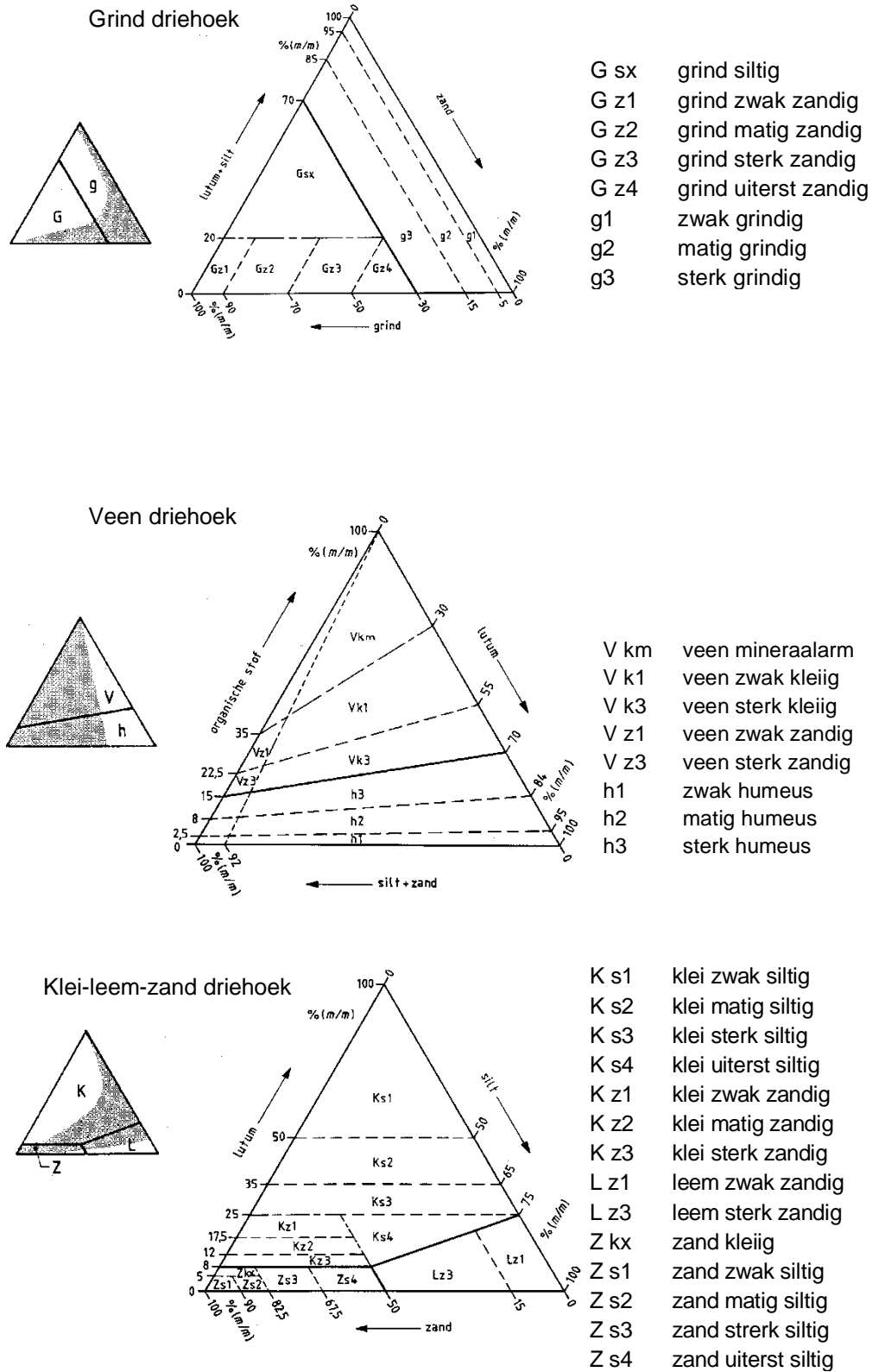
5 Figuur 3 De grondsoorten driehoeken volgens NEN 5104; de natuurlijke monsters vallen meestal in de gearceerde delen van de driehoeken (NNI, 1989).
